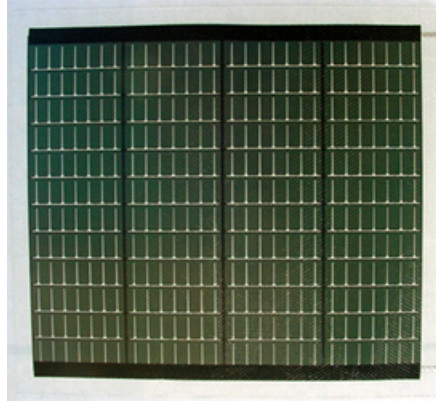
Figura 6: Paneles solares utilizados en la fuente de alimentación(PT15-300)
